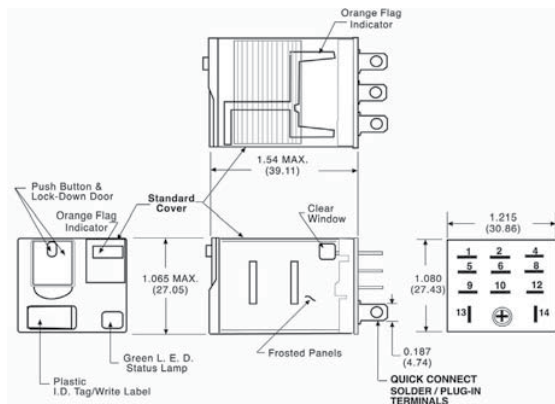
3TX7116 3PDT
