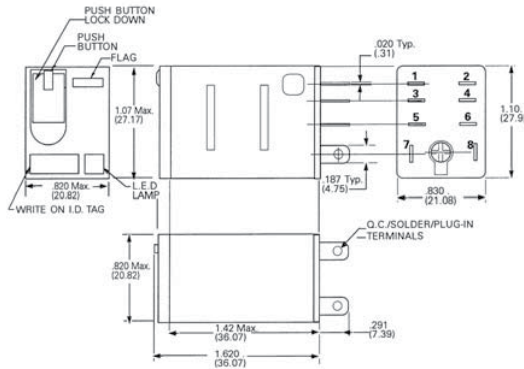
3TX7114 DPDT
