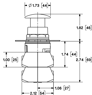
Botón pulsador momentáneo No iluminado metal
