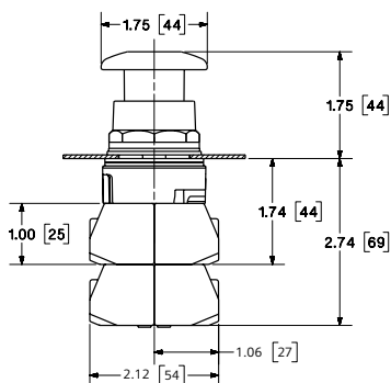
Botón hongo no iluminado Plástico 1 3/4 - Jalón
