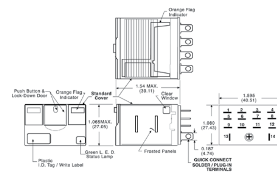
3TX7117 4PDT
