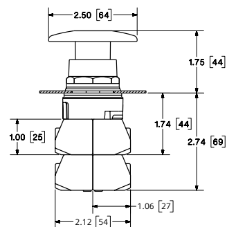
Botón hongo no iluminado Plástico 2 1/2 - Jalón
