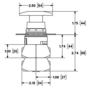
Botón pulsador hongo momentáneo no iluminado plástico 2 1/2"
