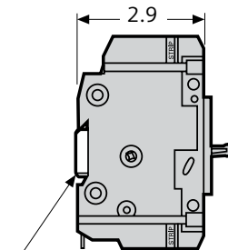
Fits 35mm DIN Rail
