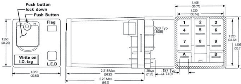
3TX7115 3PDT
