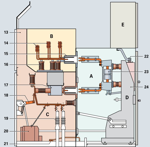
Estructura básica de la celda (ejemplo)
