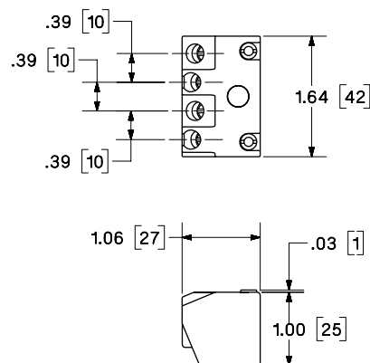
Bloques de contacto
