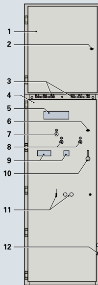
Estructura básica de la celda (ejemplo)
